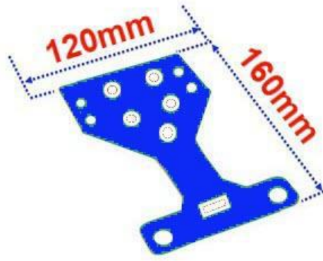
Şekil 5: Hızlı Çizgi İzleyen Robot ölçüleri
